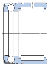
NX ( F_w \geq 10 mm)
