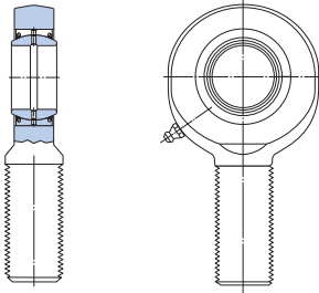
SA(L)A..ES-2RS
